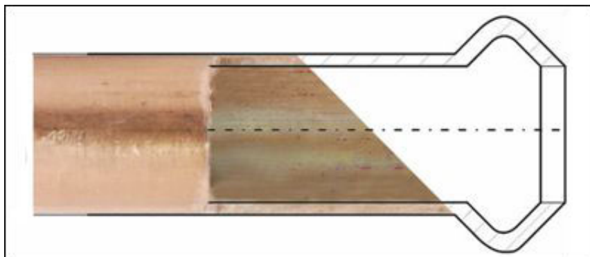
spęczniecie typu SF - grzybek
