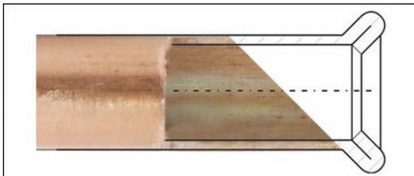
spęczniecie typu DF - kieliszek
